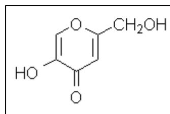
Kojic acid
